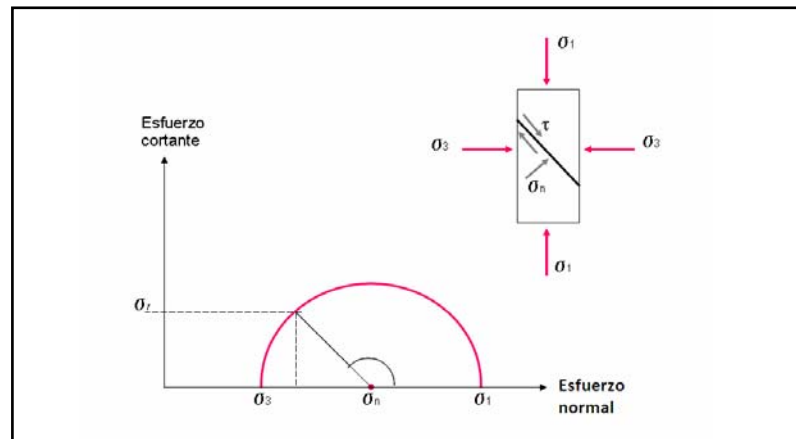
Figura 2.8. Círculo de Mohr. Fuente: González L, 2002.
