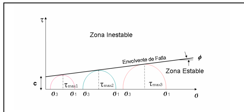
Figura 2.9. Envoltorio de falla. Fuente: González L, 2002.
