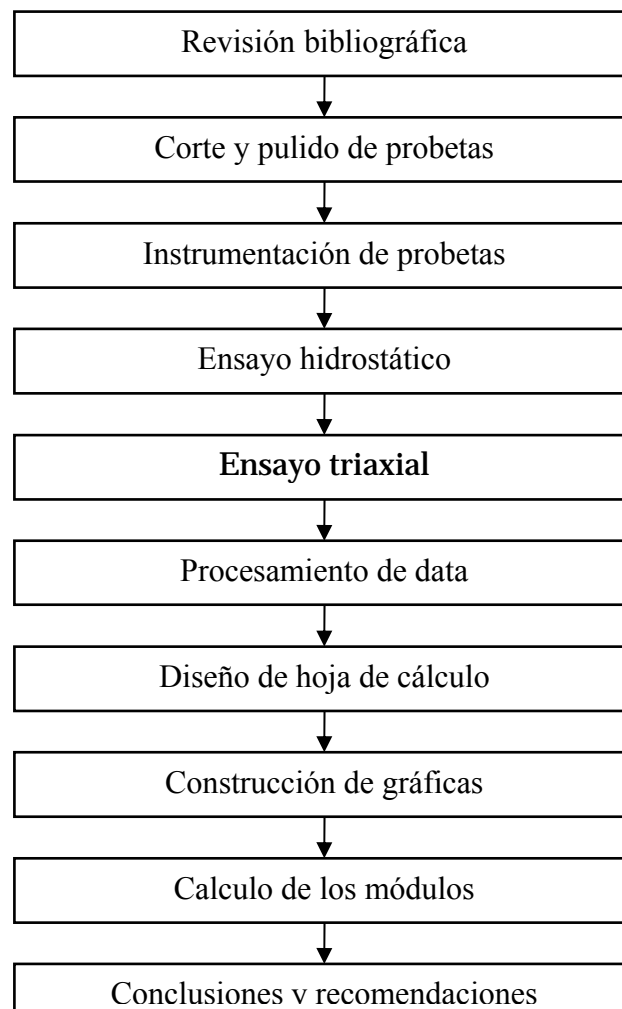
Figura 3.20. Flujograma de la metodología empleada. Fuente: Propia.
