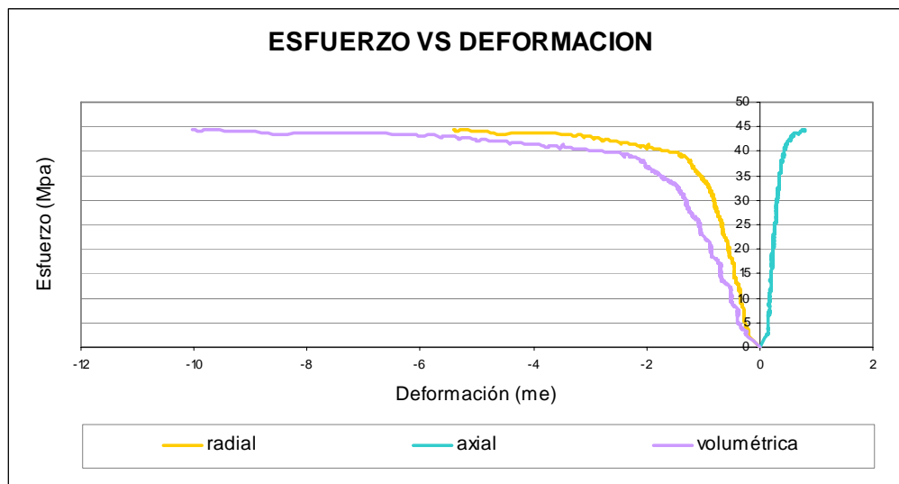
Figura 5.7. Esfuerzo vs deformación. Triaxial probeta 4. Fuente: Propia.
