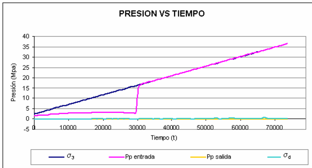
Figura 5.21. Presión vs tiempo. Ensayo muestra 15. Fuente: Propia.
