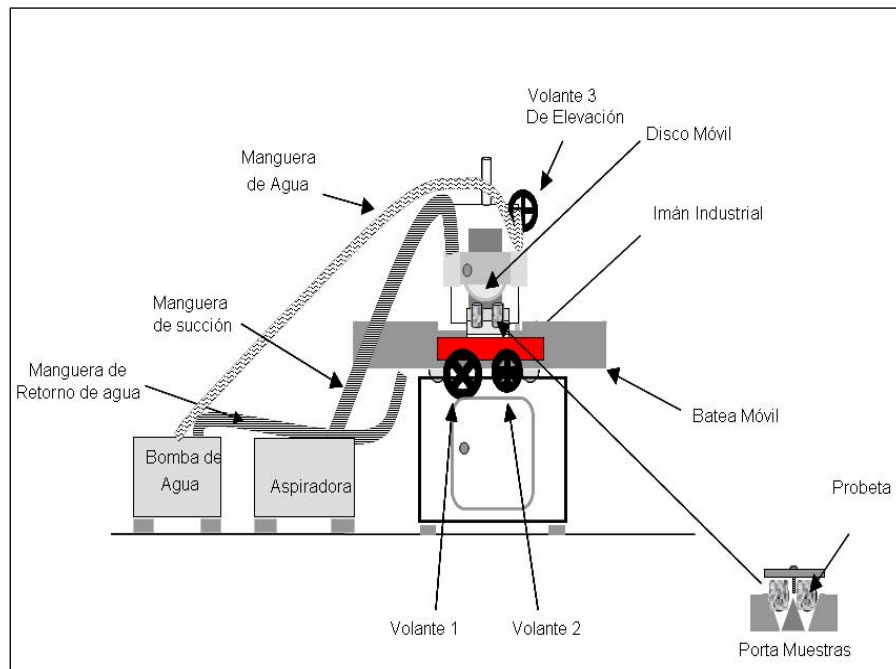
Figura 3.10. Esquema de la pulidora. Fuente: LFR, 2006.
