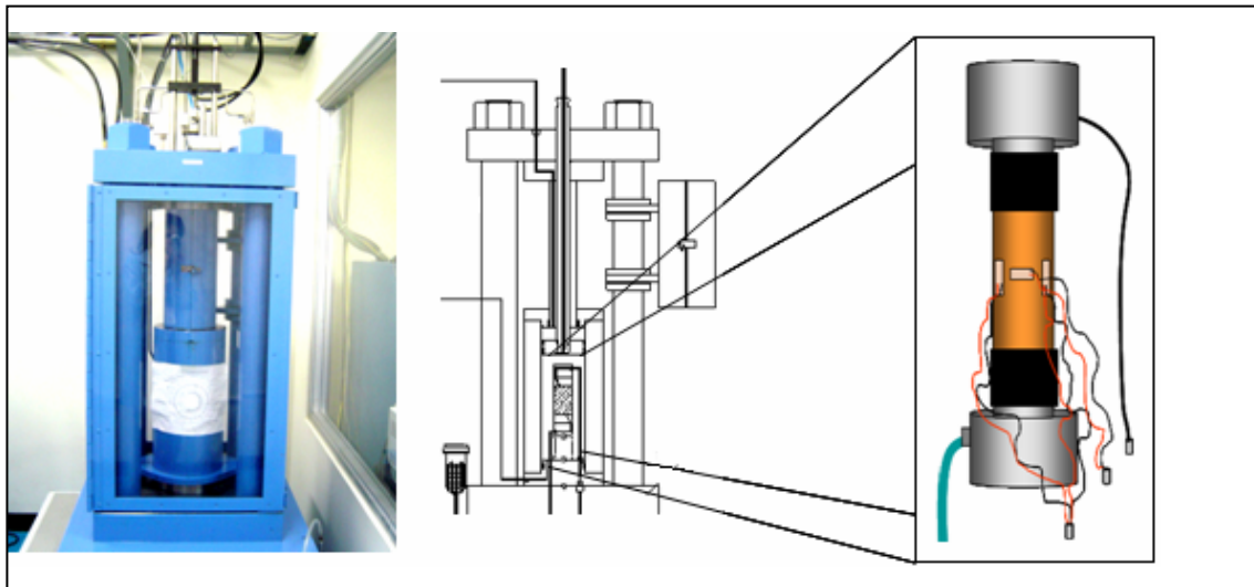
Figura 3.2. Cámara de ensayo y conexiones de sensores. Fuente: Propia, 2009.
