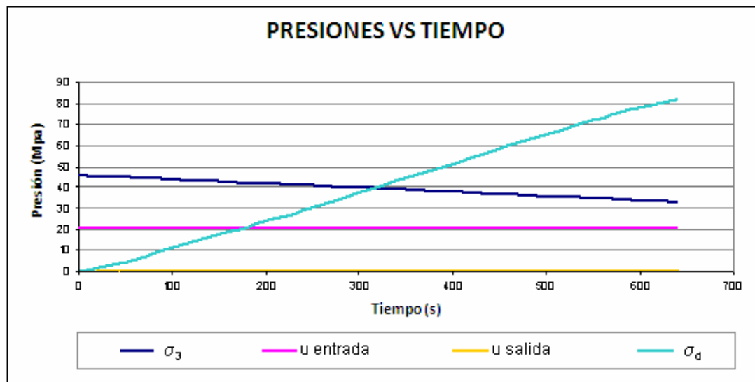
Figura 5.4. Presión vs tiempo. Triaxial probeta 3. Fuente: Propia
