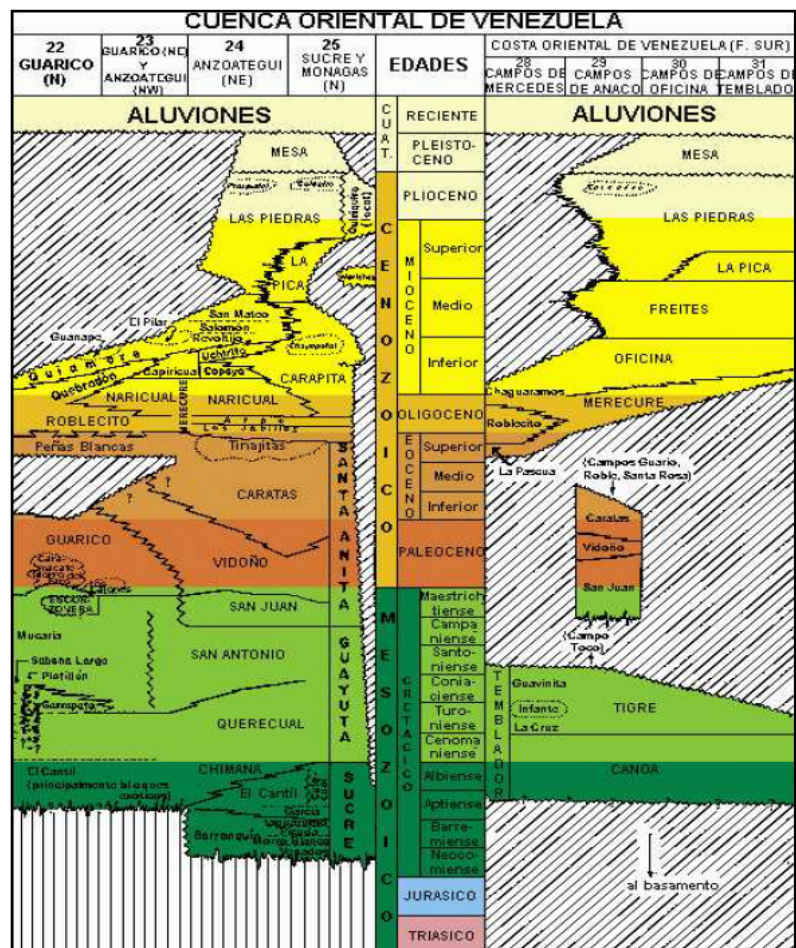
Figura. 1.3. Columna estratigráfica de la Cuenca Oriental de Venezuela. Fuente: Comité Interfilial de Estratigrafía y Nomenclatura, 1997.
