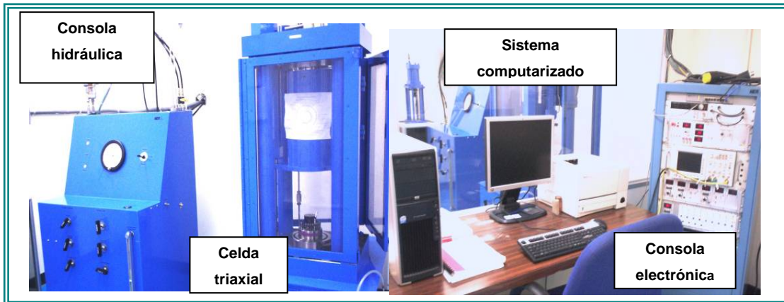
Figura 4.1. Equipo Autolab2000.Fuente: Propia
