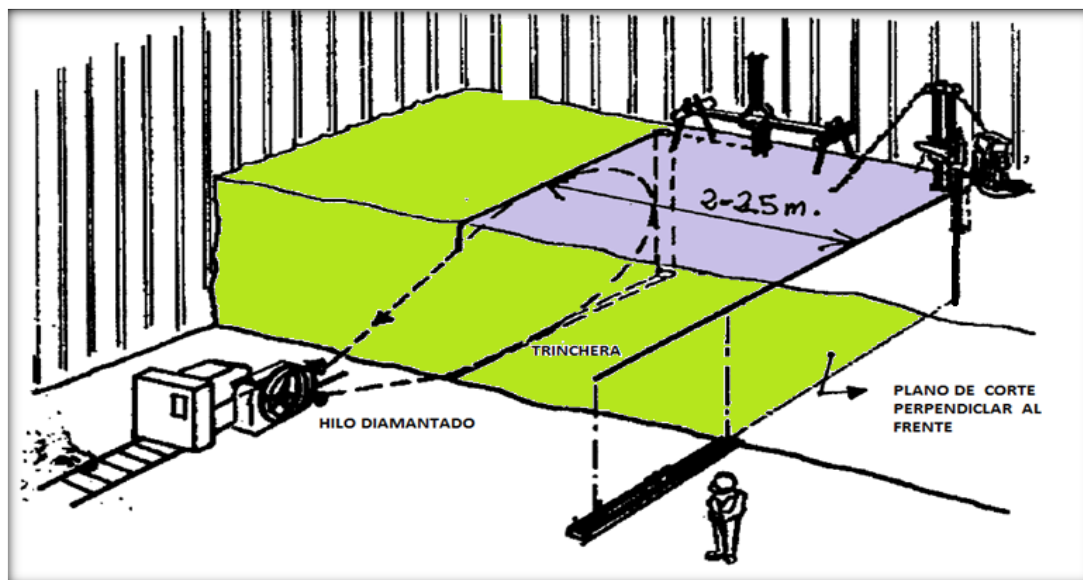
Figura 3.2. Apertura de una trinchera utilizando un equipo de cable diamantado y perforación
