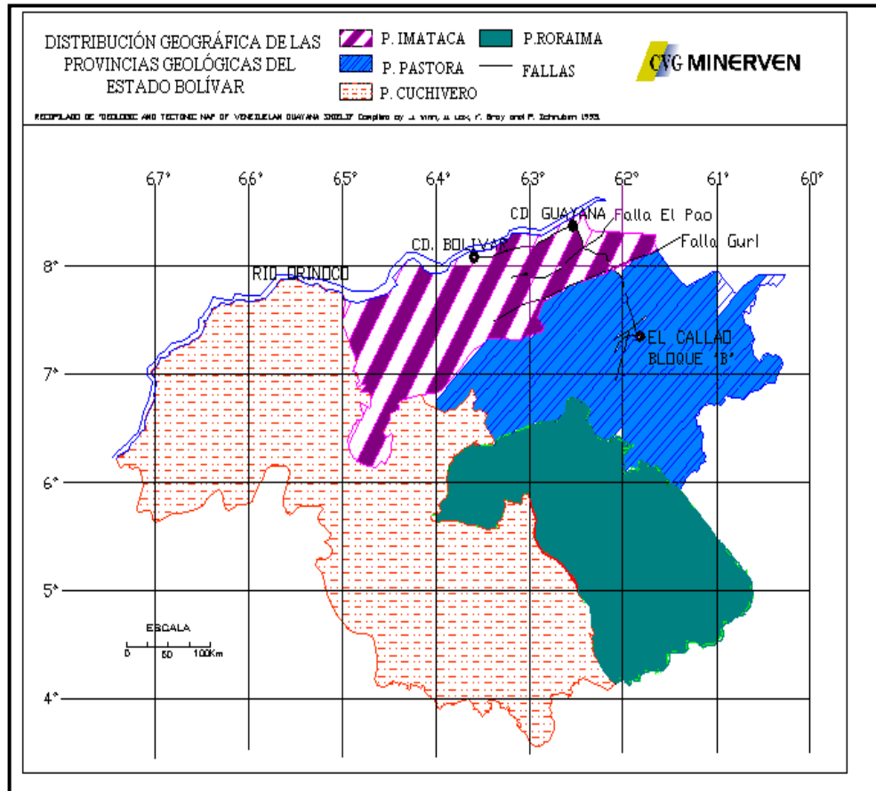
Figura 2.7 Provincias Geológicas del estado Bolívar. (C.V.G. Minerven)
