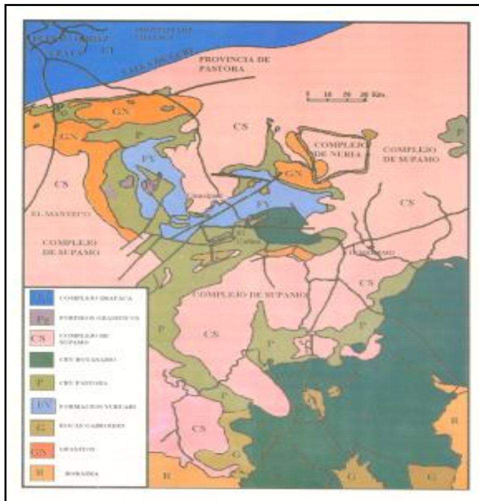
Figura 2.5 Extensión de la Provincia de Pastora en la parte Oriental del Escudo de Guayana (Tomado de Mendoza, 2000)
