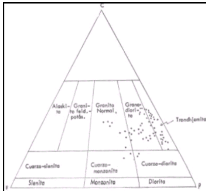
Figura 2.6 Complejo de Supamo Triangulo (C.F.P.) Cuarzo-feldespato potásico-Plagioclasa (Menéndez, 1972)
