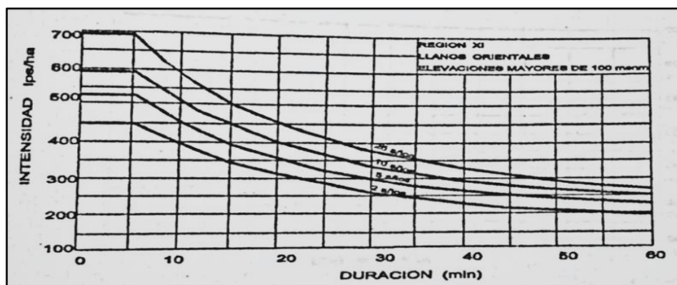
Figura 5.12 Curva IDF para la Región XI (Llanos orientales con elevaciones superiores a los 100 msnm), (Camacho, 2004).
