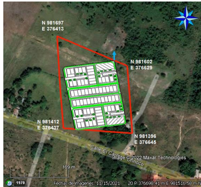
Figura 5.8 Punto de drenaje del urbanismo hacia el norte (flecha azul).
