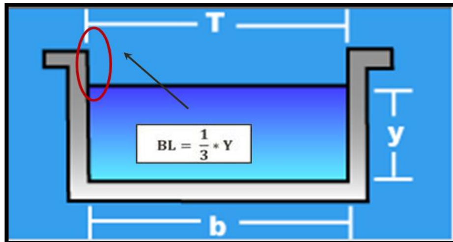
Figura 6.1 Esquema de la sección transversal de la torrentera.
