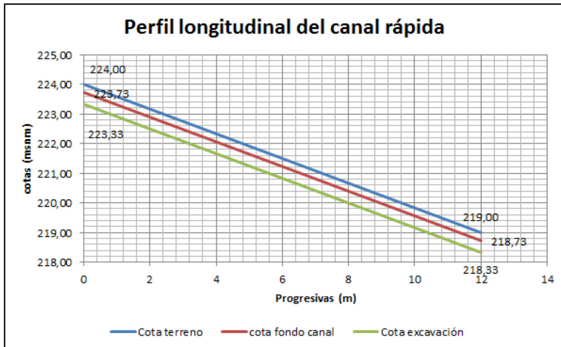
Figura 5.15 Perfil longitudinal de la rápida sin disipación.
