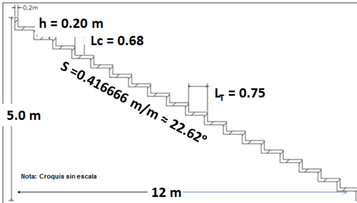
Figura 6.2 Perfil longitudinal típico de la rápida escalonada.
