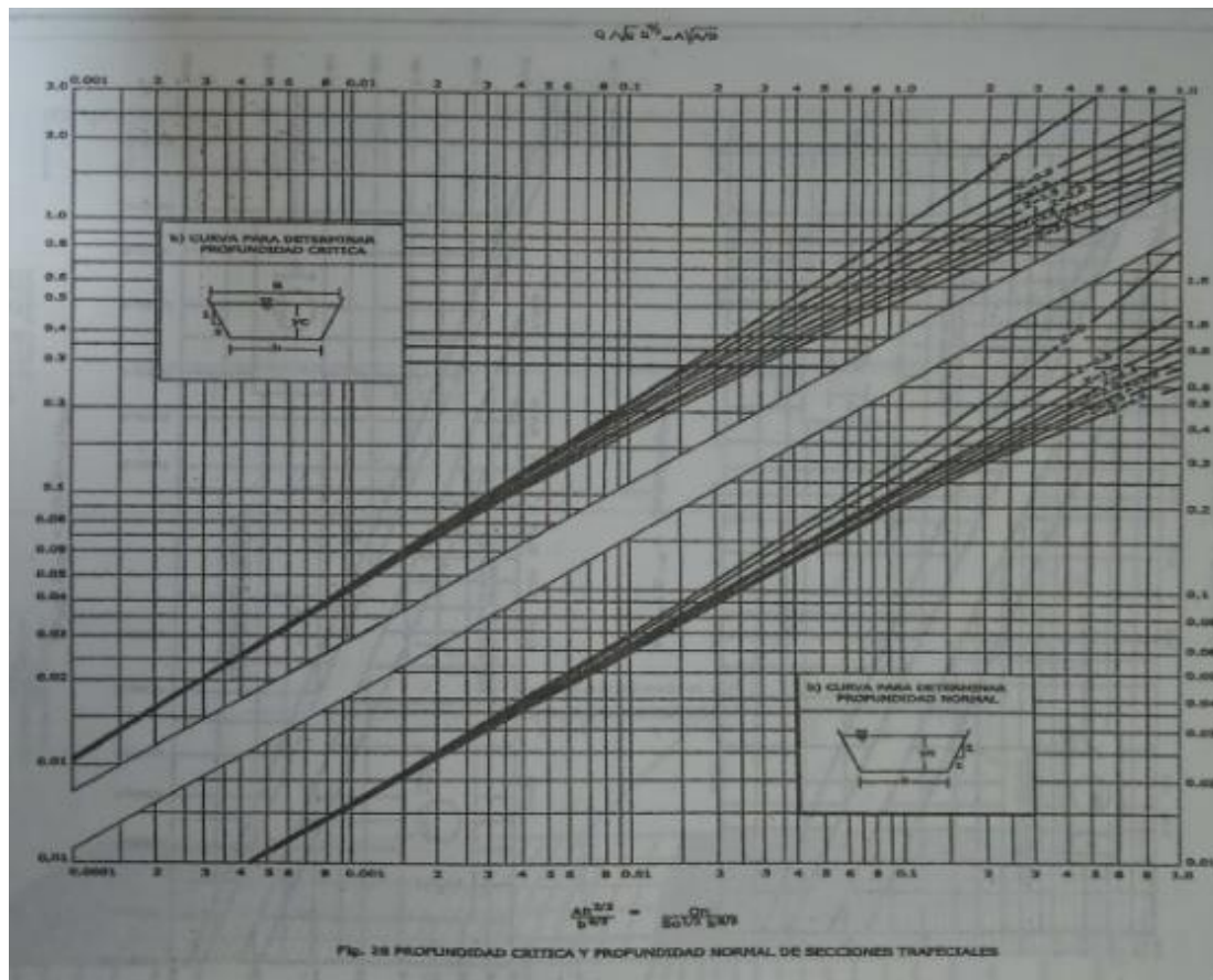
A.2 Estimación de profundidad normal y profundidad crítica en canales rectangulares y trapeziales (Camacho, 2004).
