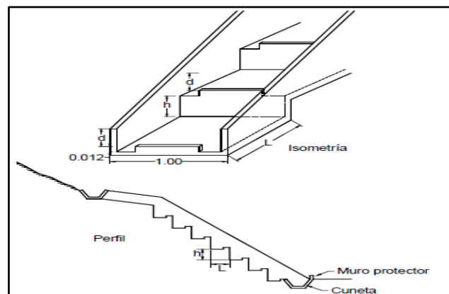
Figura 3.3 Torrentera en gradería con bloques en el fondo (Aristizabal et al, 2013).
