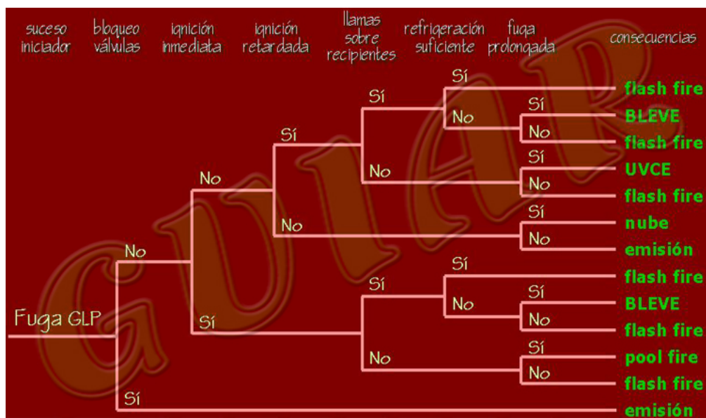
Gráfico 5. Árbol de Sucesos para Fuga de GLP en Zona Próxima a Depósitos de Almacenamiento.
