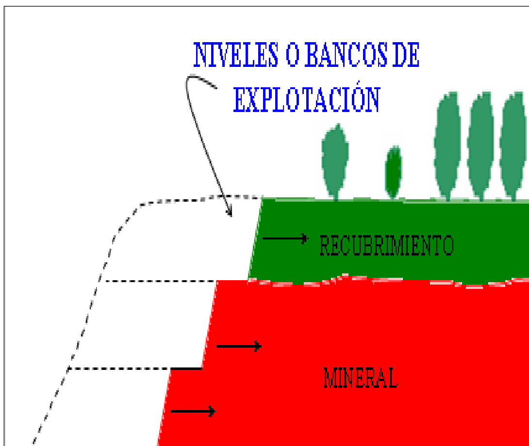
Figura 5.3. Método de explotación en tiras o " Stripping Mine ". (Chacón, E. 1997).
