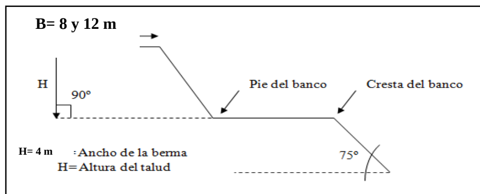
Figura 5.2 Parámetros geométricos del desarrollo minero. (Chacón, E. 1997).
