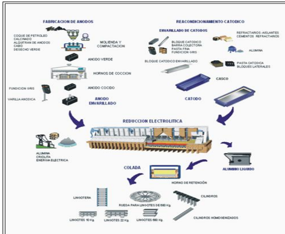
Figura 3.1 Proceso de obtención del aluminio. (Chacón, M. 2008)
