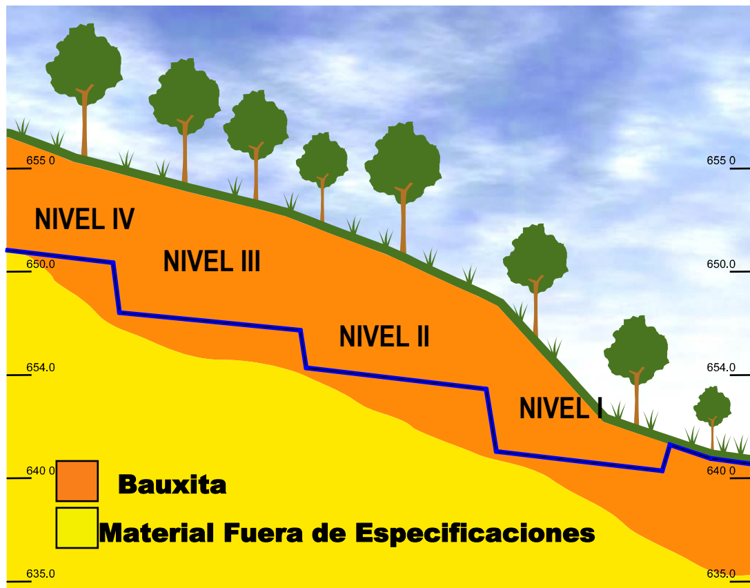
Figura 5.4 Método de explotación combinado “ Stripping Mine ”. (Chacón, E. 1997).
