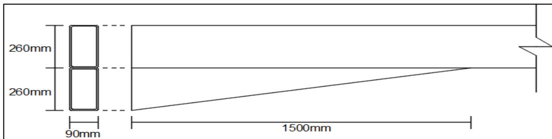
Ilustración 57: Detalle de cartela para Perfil Conduven 260x90x5.5mm Fuente: Autor (2020)
