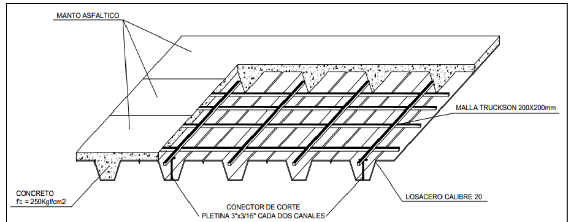
Ilustración 72: Losacero empleada en techo Nivel N+7.25. Fuente: Autor (2020)
