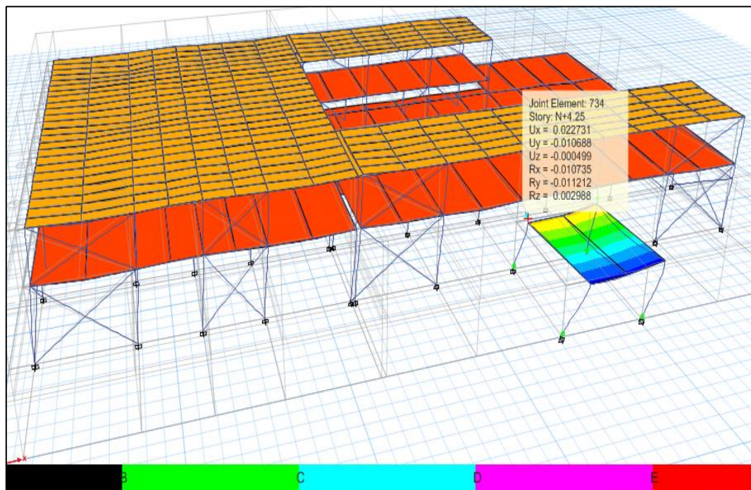
Ilustración 81: Aparición de rotula plástica color azul celeste en D1 N+3.00
