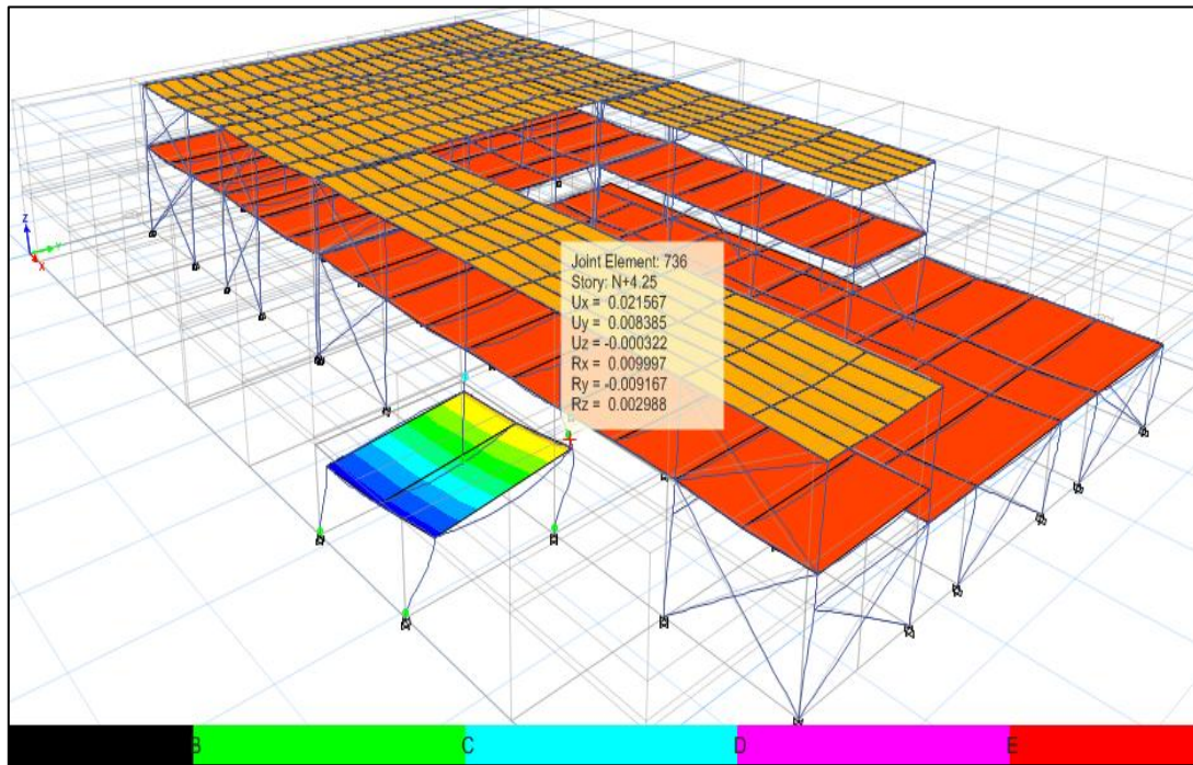
Ilustración 80: Aparición de rotula plástica color verde en C0, C1, D0, D1 Nivel planta, y C1 N+3.00
