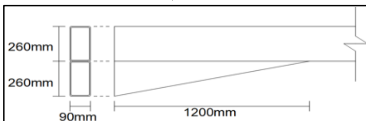
Ilustración 59: Detalle de cartela para Perfil Conduven 260x90x5.5mm, en pórticos de 3.13mL Fuente: Autor (2020)
