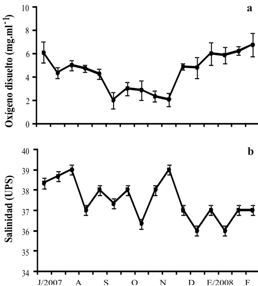
Figura 8. Concentración de oxígeno disuelto (a) y salinidad (b) en la ensenada de Turpialito, golfo de Cariaco, estado Sucre, Venezuela.
